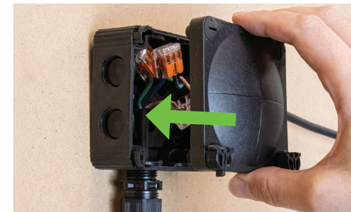
12 Connect WISKA® COMBI® 308 lid
